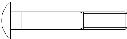
M10*65 - 4PCS
